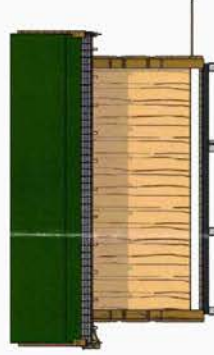
Vest Fasade
