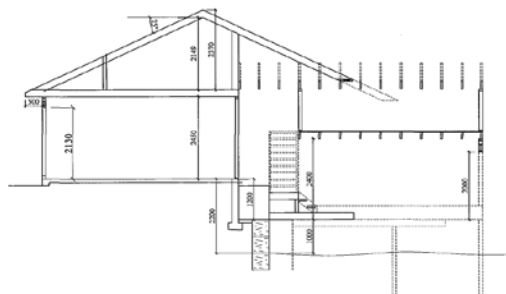
Snitt B-B
